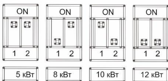
Рис. 9. Положение рычагов переключателя мощности.
