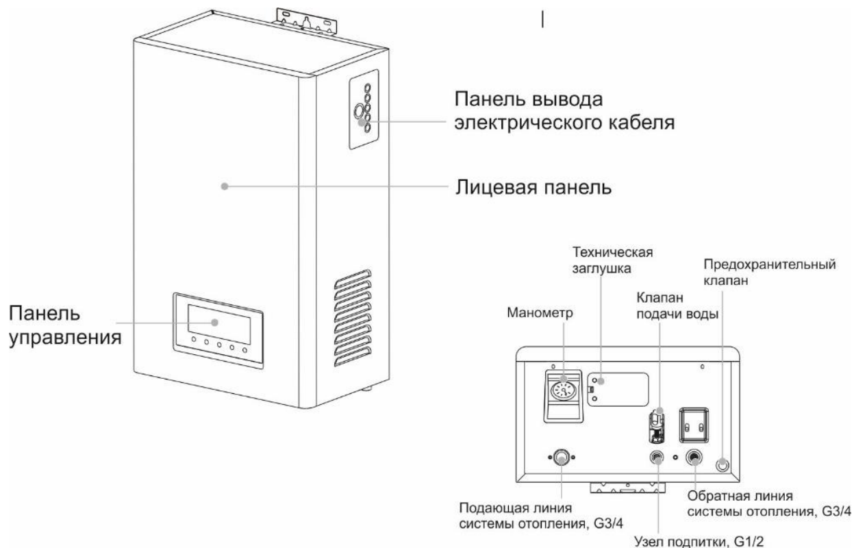
Рис. 1. Конструкция изделия
