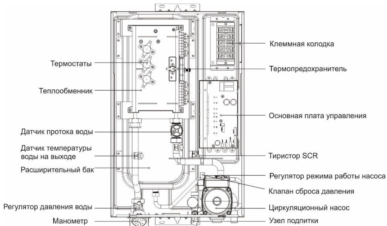
Рис. 2. Схема внутреннего устройства изделия
