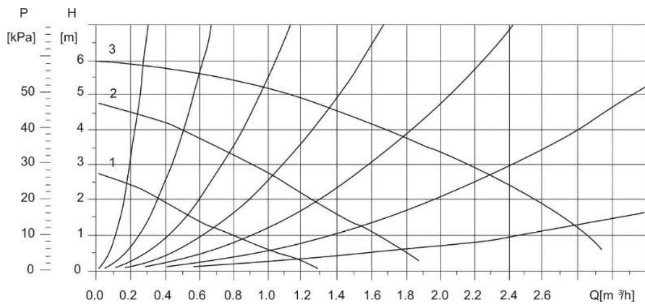
Рис. 14. Кривая характеристик давления насоса
