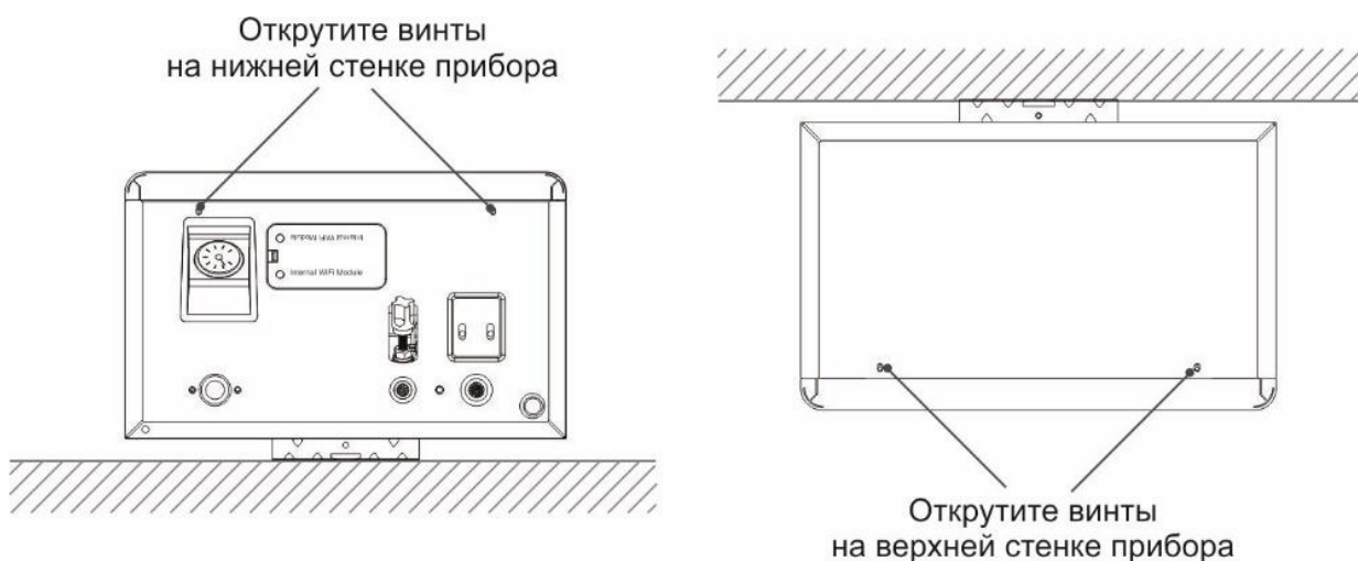
Рис. 8. Демонтаж лицевой панели
