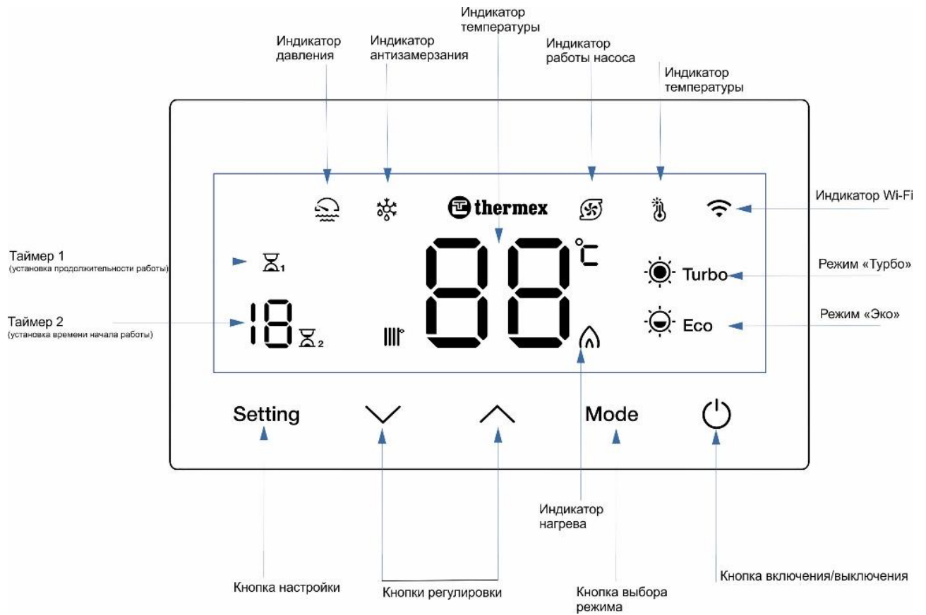
Рис. 3. Панель управления
