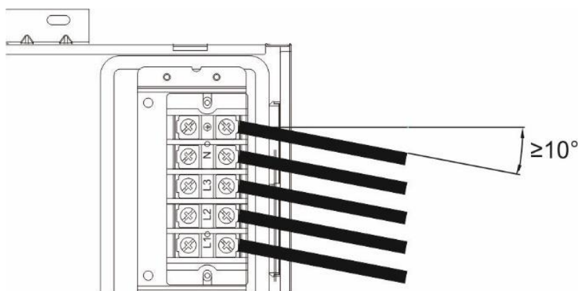
Рис. 13. Расположение сетевого кабеля
