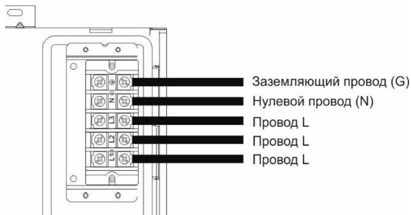
Рис 12. Трехфазное подключение прибора
