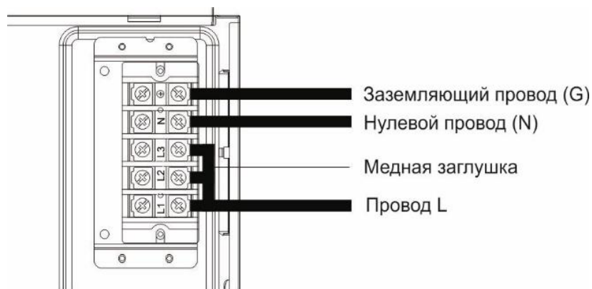
Рис 11. Однофазное подключение прибора
