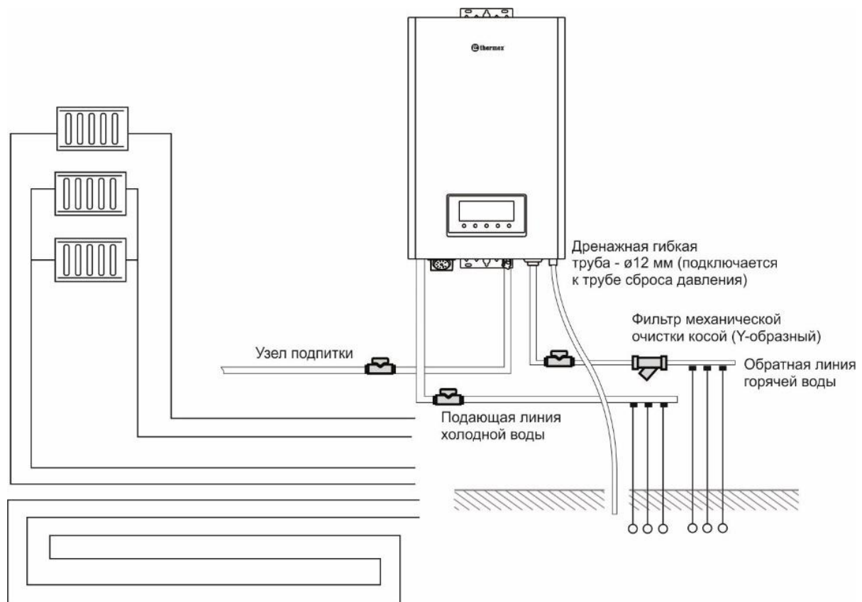
Рис. 4. Схема подключения труб
