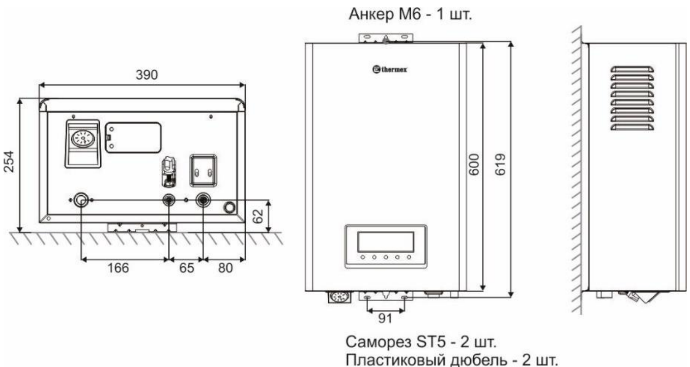
Рис. 6. Монтажные размеры
