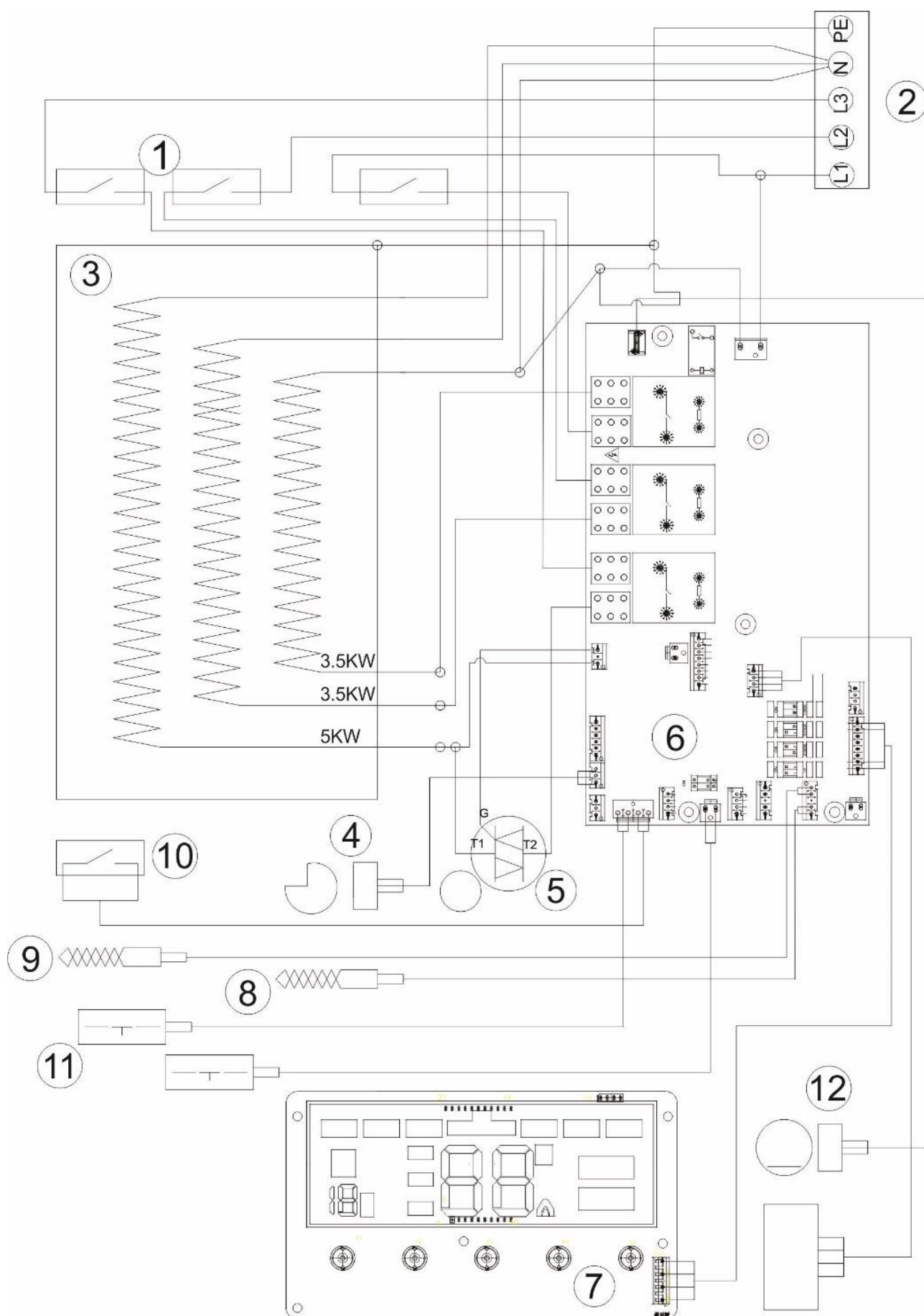
Рис. 15. Электрическая схема THERMEX Grizzly 5-12 Wi-Fi
