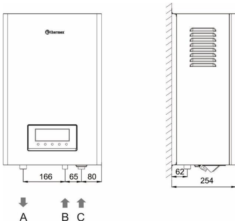
Рис. 7. Присоединительные размеры
